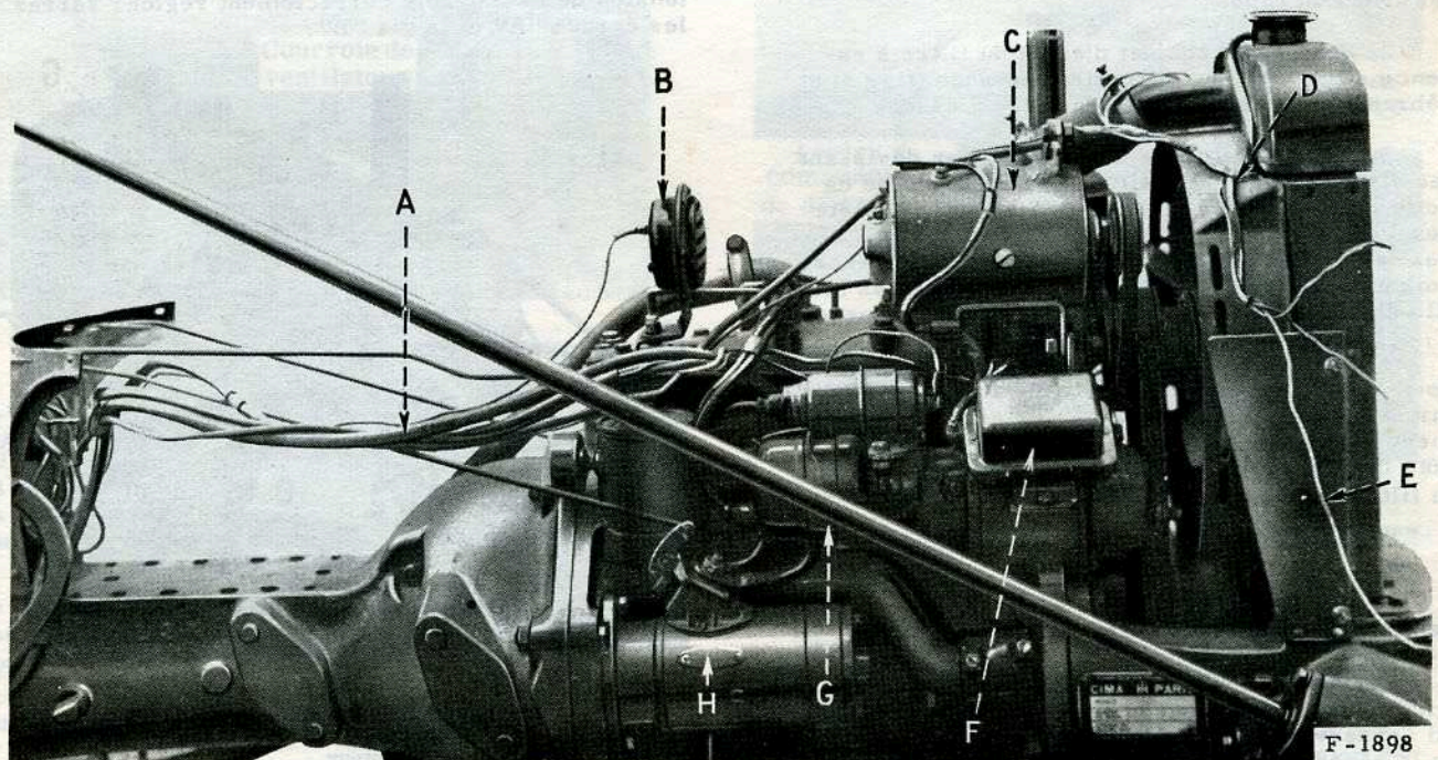
Figure 41 - Démarreur, génératrice, régulateur de tension et câbles
