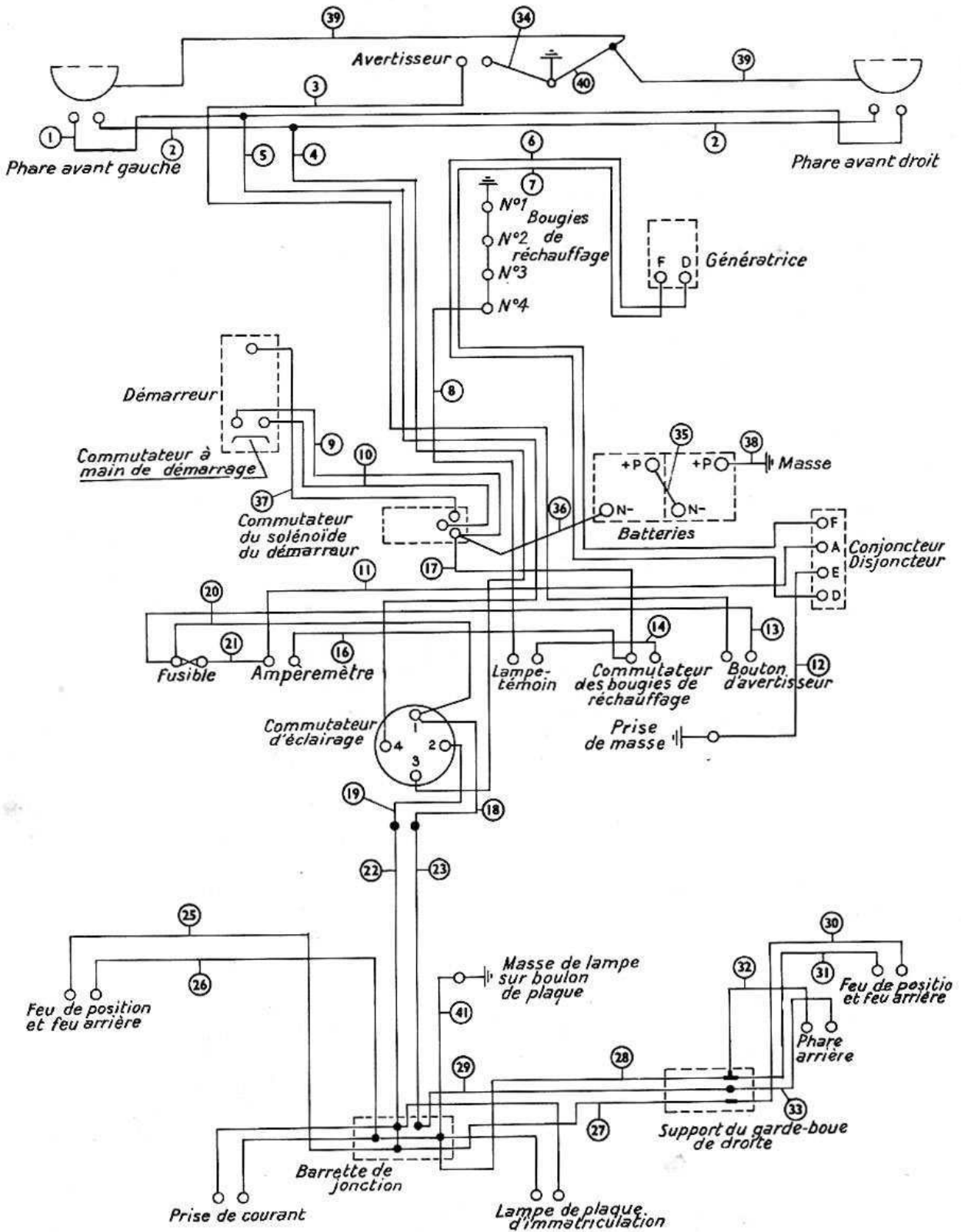
Fig. 44 - Schéma de câblage
